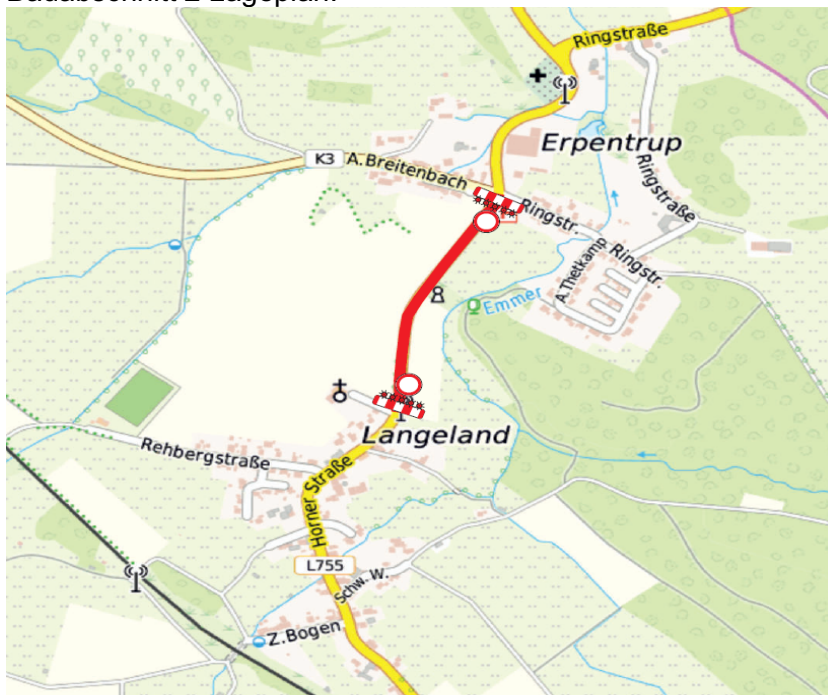
Bauabschnitt 2 Lageplan:
